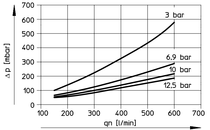
MS6-LDM1-...-P30
