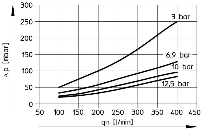
MS6-LDM1-...-P40
